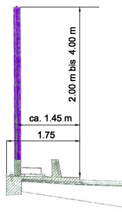
Querschnitt Brücke
