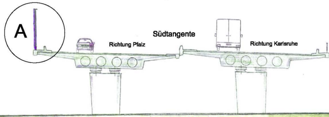
Brückenquerschnitt
